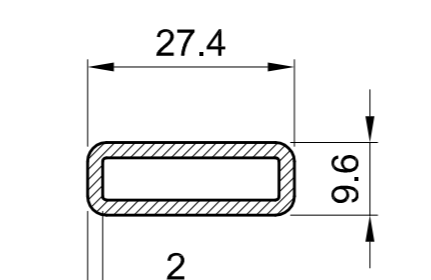
655 010 27 / 10 / 2 mm galvanized steel Ix= 0,16 cm 4 Iy= 0,95 cm 4 Insert: 652 010
