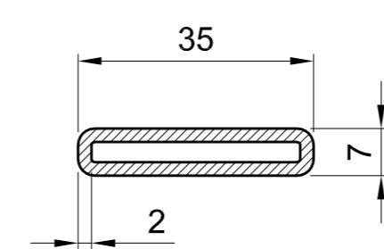
655 020 35 / 7 / 2 mm galvanized steel Ix= 0,09 cm 4 Iy= 1,61 cm 4 Insert: 650 020, 650 030, 650 040, 650 050
